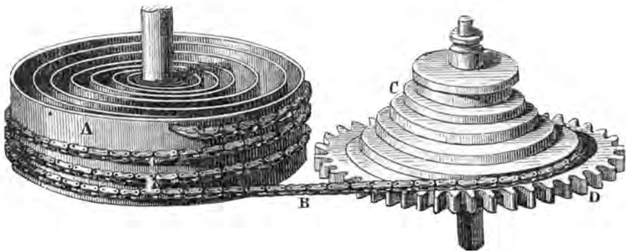
Abb. 2: Schnecke und Trommel (aus: Franz Reuleaux: Erfindung und Herstellung der Uhren, in: Das Buch der Gewerbe, Erfindungen und Industrien, Leipzig 1900, Bd. 6, S. 598). Während die Feder abläuft, kompensiert der größere Hebelarm die schwächer werdende Kraft der Feder und hält so die Antriebskraft konstant.
